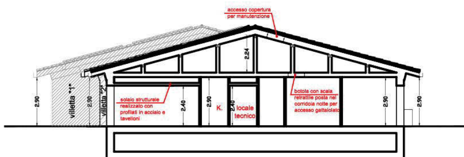
SEZIONE
